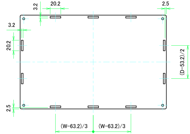
上カバー裏面 / Top cover Backside
