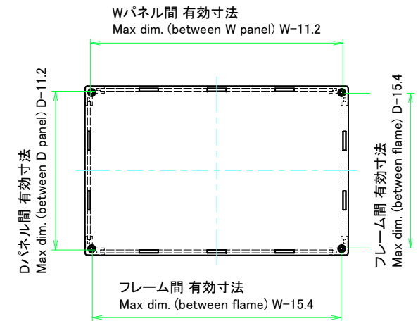
下カバー / Bottom cover
